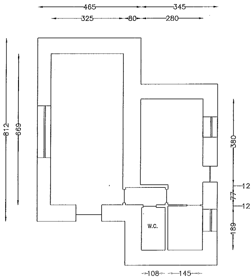
PIANTA P.TERRA
