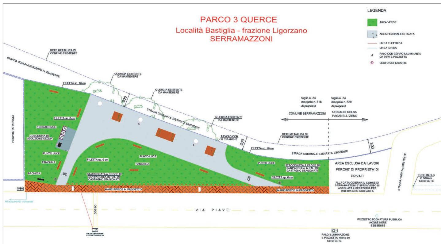
Schizzo del progetto
